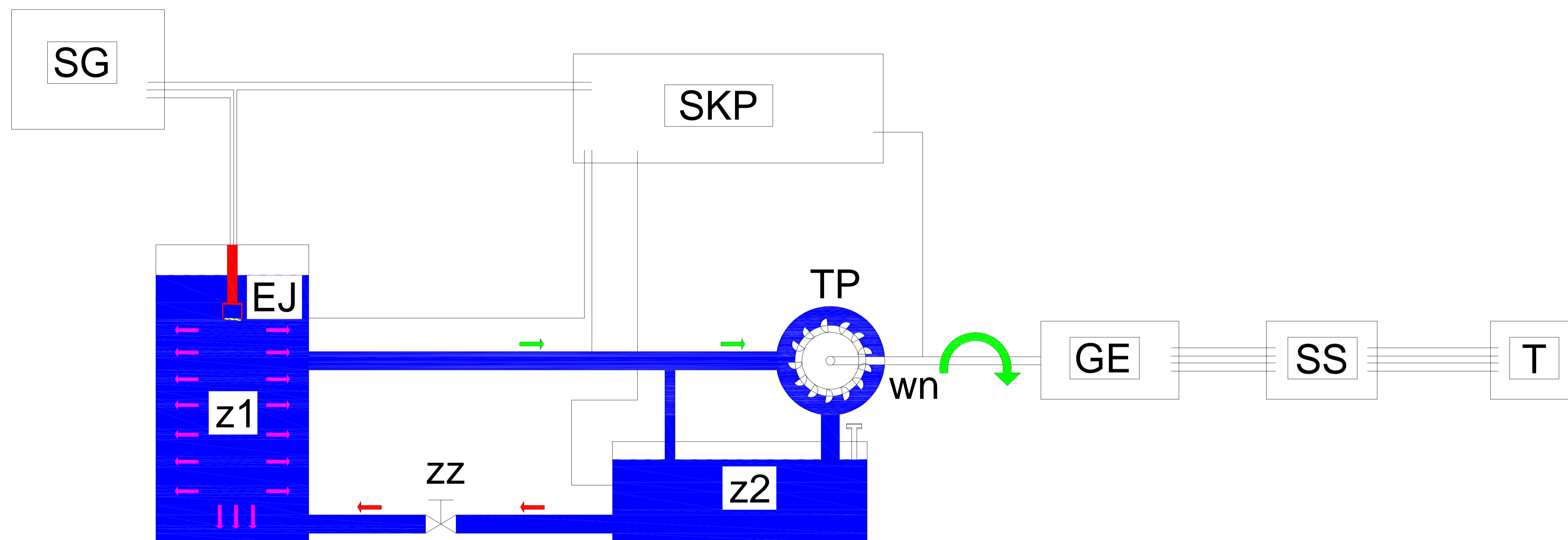
SG- sterownik generatora iskry; SKP- stacja kontrolno- pomiarowa; GE- generator elektryczny; SS- szafa sterująca; T- transformator; z1- zbiornik główny, z2- zbiornik pomocniczy; EJ- elektroda Jutkina; TP- Turbina Peltona; wn- wał napędowy generatora; ZZ- zawór zwrotny.
